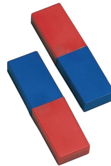
bar magnet
