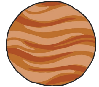
Jupiter
